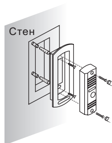
(1) Монтаж заподлицо
