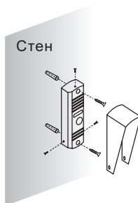
(2) Поверхностный монтаж
